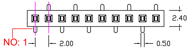
TYPE 1 正脚位
