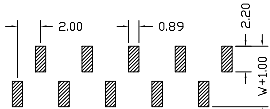
TYPE 1 正脚位
