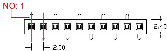
TYPE 2 反脚位
