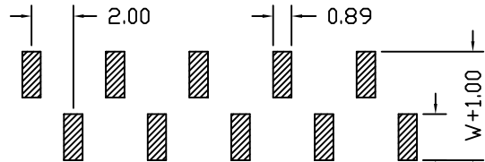
TYPE 2 反脚位
