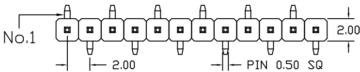
TYPE 2 (反脚位)
