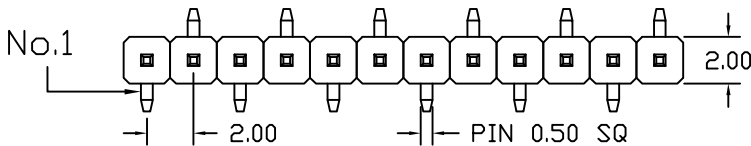
TYPE 1 (正脚位)
