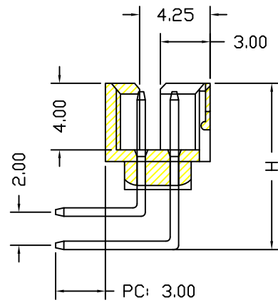
SEC A-A SCALE 1:1
