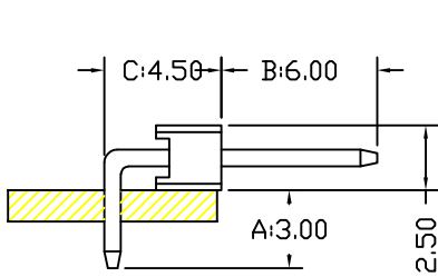
R1 Type (顶弯)
